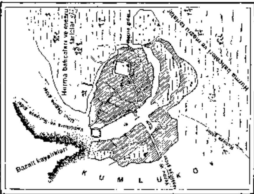
Medine planı
